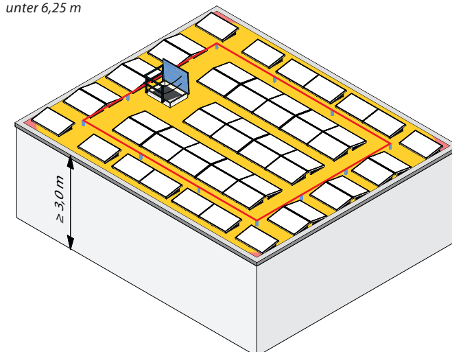
Abb. 8: Ausstattungskategorie 2: Rückhaltesystem bei ganzflächigen Solaranlagen
