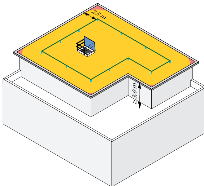
Abb. 7: Ausstattungskategorie 2: Rückhaltesystem zwingend bei geringem Sturzraum einsetzen, z. B. bei Attikaterassen oder bei Anbauten mit Höhen unter 6,25 m
