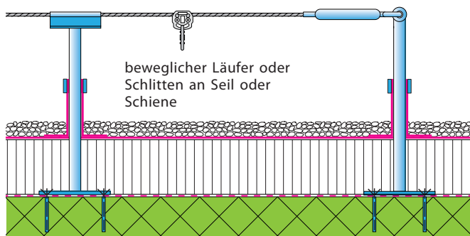
Abb. 5: Ausstattungskategorie 2: permanentes horizontales Seilsystem mit Spannfeder, direkt in Stahlbeton verankert
